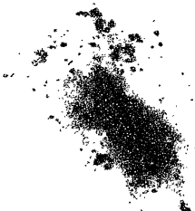
NGC 4449
